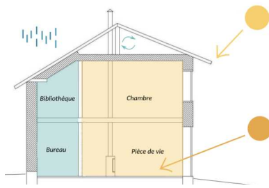
Coupe Nord Sud d'une maison bioclimatique
