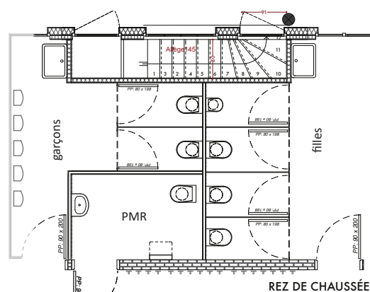
plan des TS et de la salle de compostage
