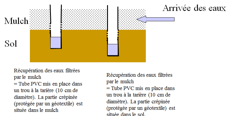
Figure 1 : Prélèvement en filière non drainée par piézomètre
