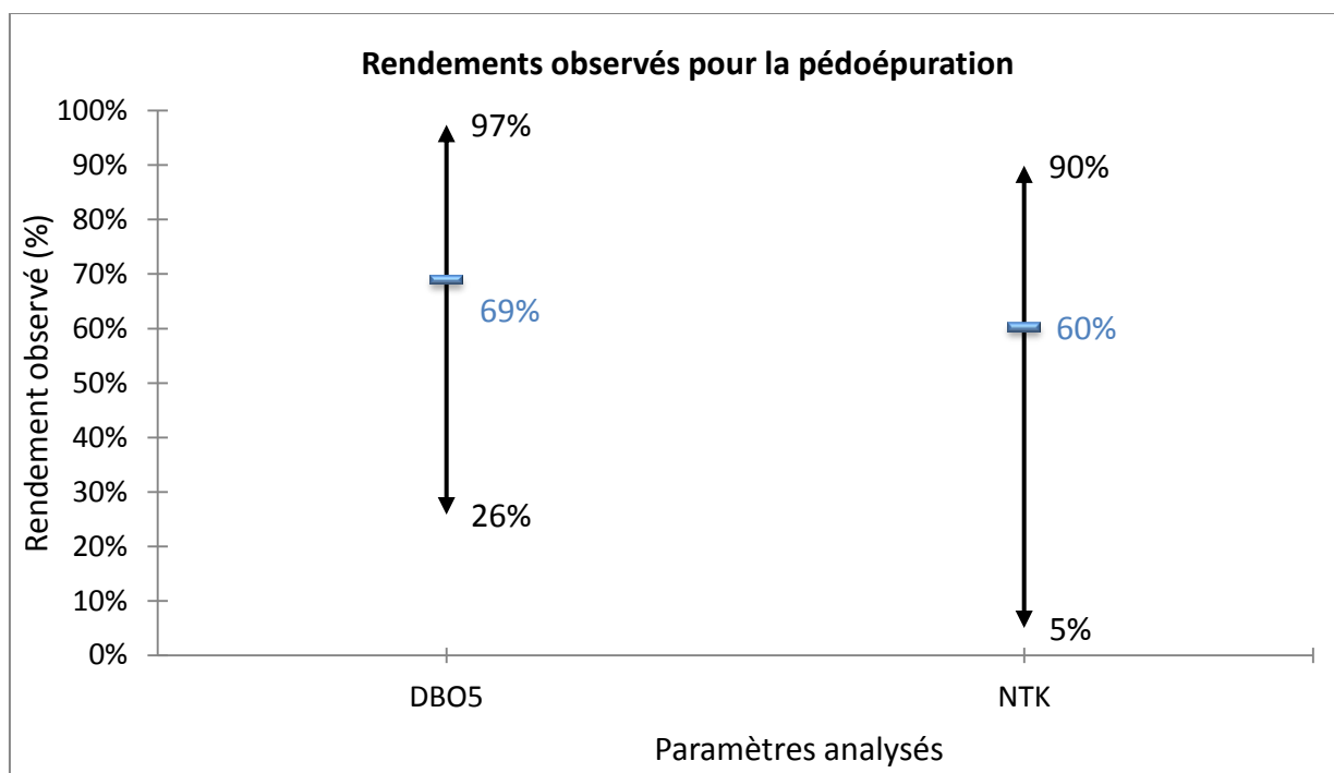
Figure 24: Rendements observés pour la pédéoépuración
