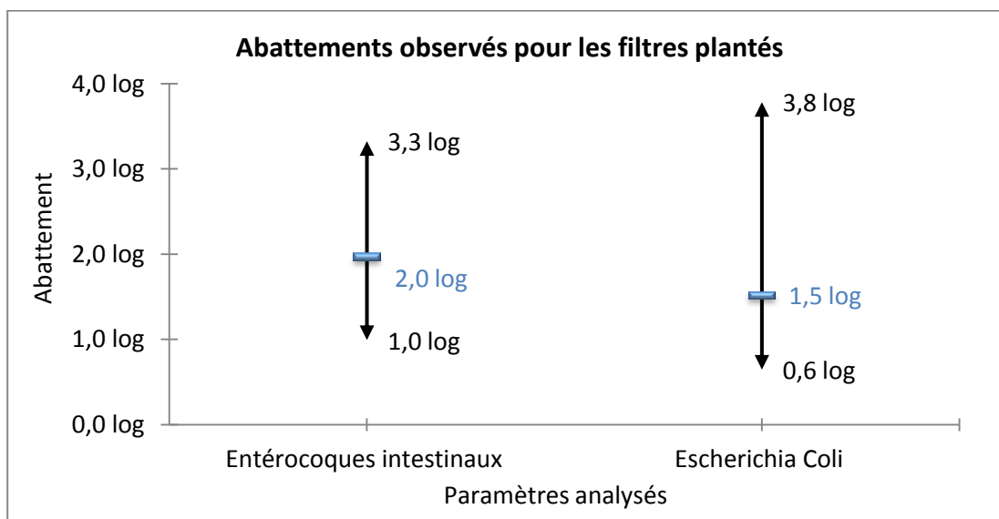
Figure 20: Abattements observés pour les filtres plantés
