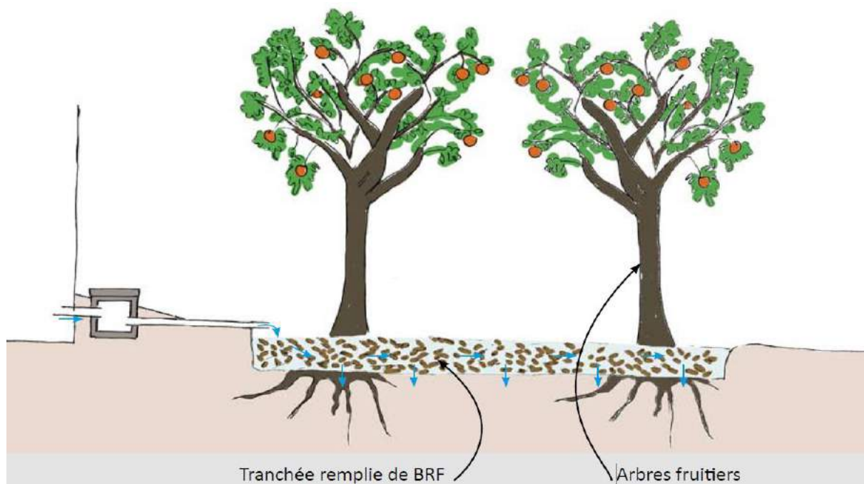
Figure 8 Coupe schématique d'une pédéoéparation (Source [6])
