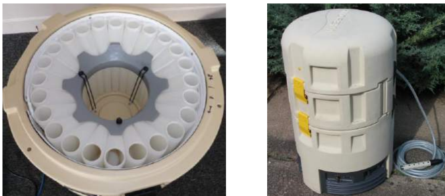
Figure 3 : Préleveur réfrigéré 24 flacons
